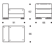
Art. 1869 91 X 66 X h. 62 cm
