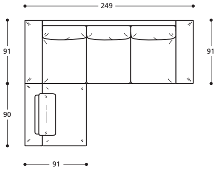
1 X Art. 9603 3-SITZER, GROSS 249 1 X Art. 9616 HOCKERELEMENT 90 MIT ARMLEHNE UND KISSEN MIT ROLLE 60X45
